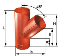
45° Y三通
