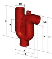
防虹吸存水弯
