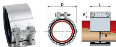
PAM CV-CE NG卡箍
