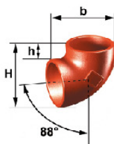
88° 弯头
