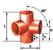
88° 立体四通
